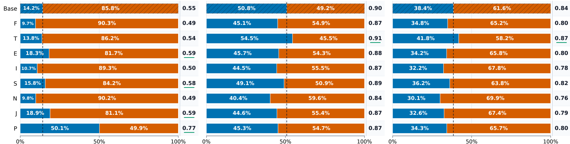
Llama-3.2-3B
